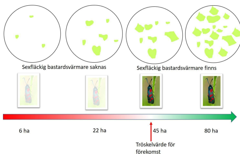
Figur Sexfläckig bastardsvärmare (fig 16 Landskap i balans). Schematisk beskrivning av tröskelvärden för hur mycket av livsmiljö som måste finnas för att en art ska kunna överleva. Exemplet här beskriver tröskelvärdet för sexfläckig bastardsvärmare som kräver att 45 hektar av torra och friska naturliga gräsmarker ska finnas inom 25 km 2 för att den ska kunna överleva.
